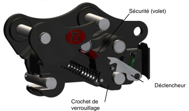
Coupe partielle du coupleur TRIGGER System® – Système verrouillé
